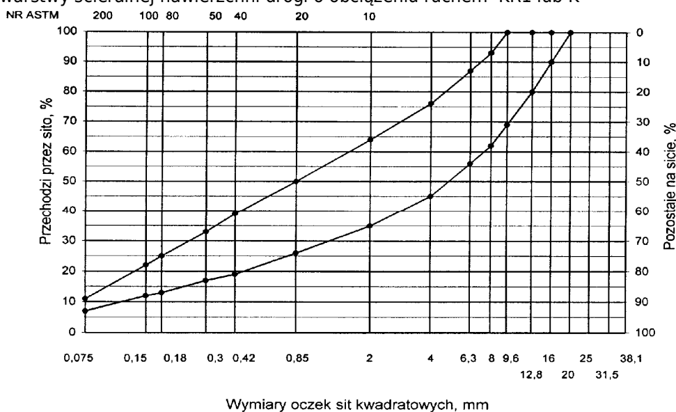
Rys. 2. Krzywe graniczne uziarnienia mieszanki mineralnej BA od 0 do 16mm, od 0 do 12,8 mm do warstwy ścieralnej nawierzchni drogi o obciążeniu ruchem KR1 lub K
